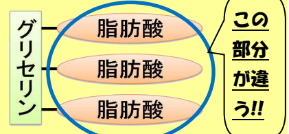
トリアシルグリセロール
